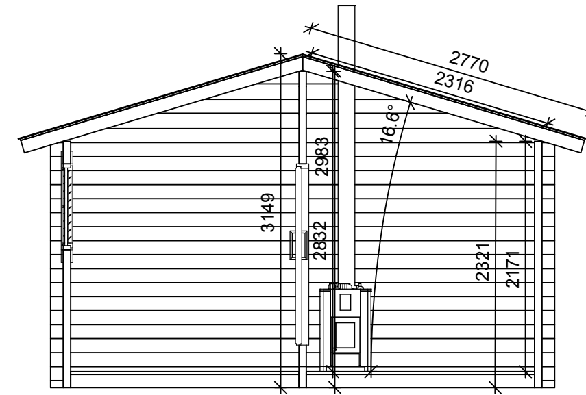
Leikkaus A-A
